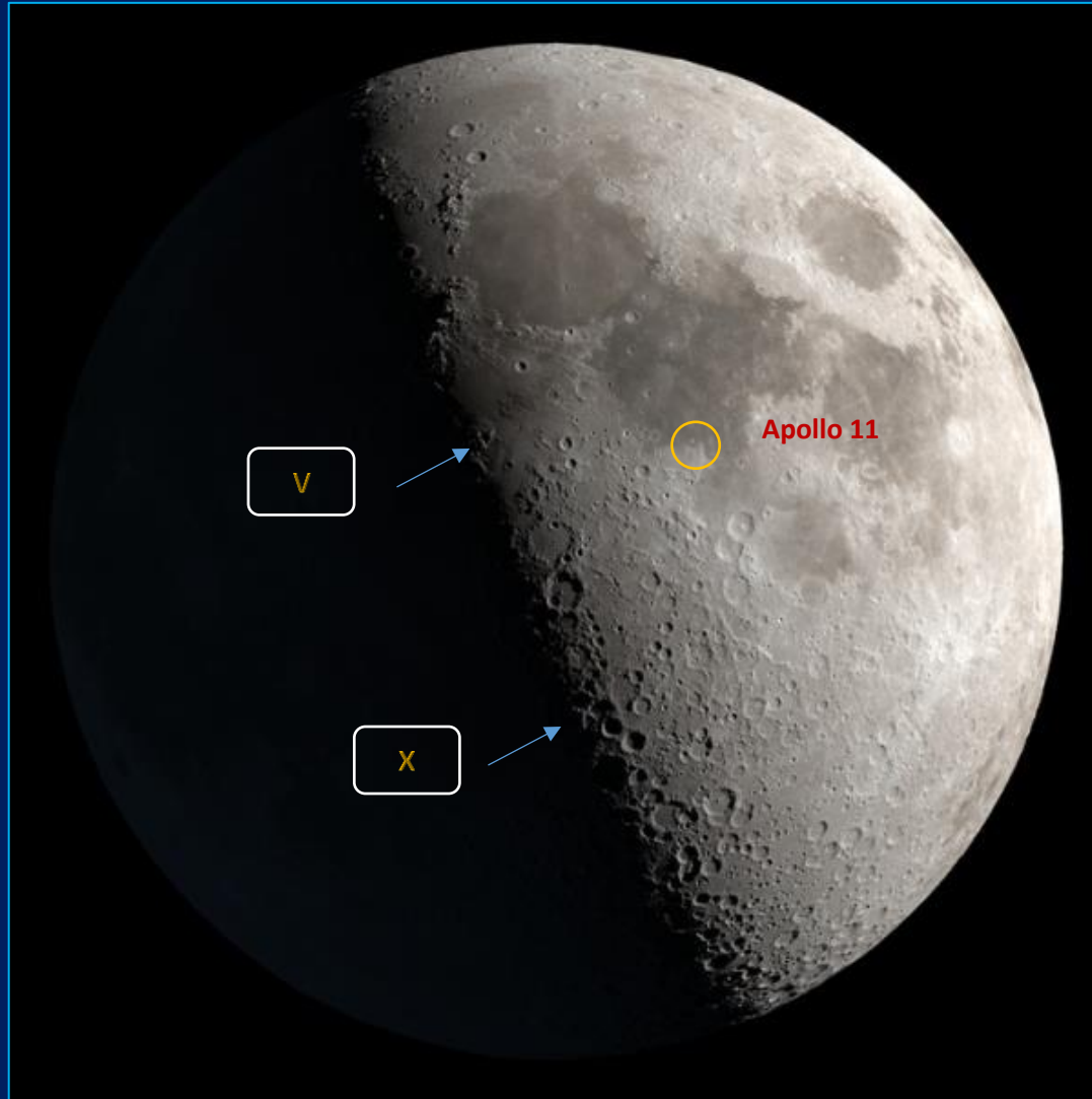
Aspect de la Lune le 09 juillet vers 20h
