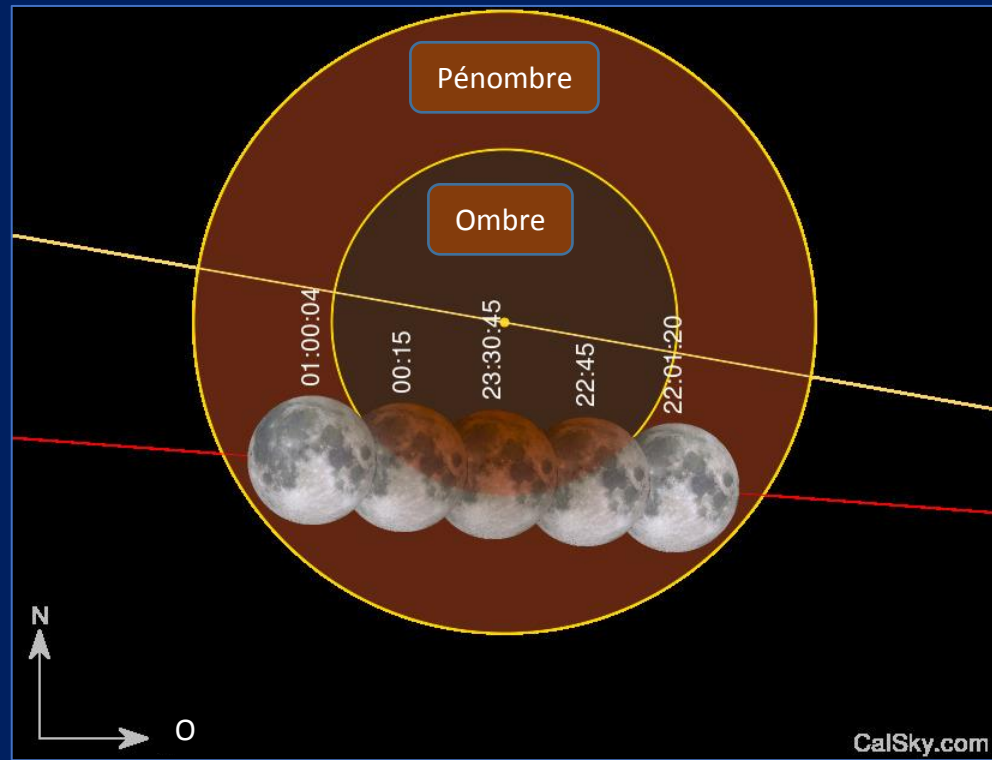
La Lune infuse dans l'ombre de la Terre. Nuit du 16 au 17 juillet 2019
