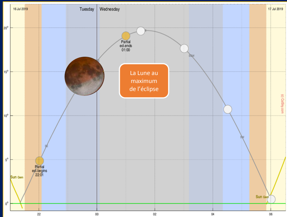
Hauteur de la Lune en fonction des différentes phases de l'éclipse partielle. (Il s'agit également de la plus basse Pleine Lune de l'année 2019)
